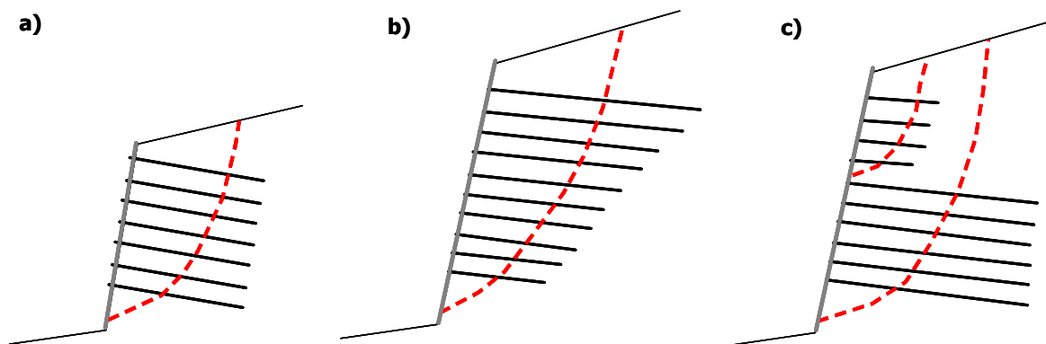
Fig. 93 – Varianti progettuali di chiodature in relazione al contesto di intervento.
