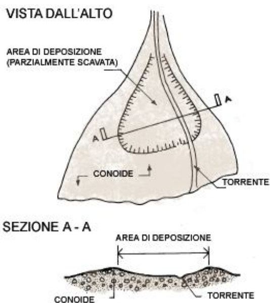
Fig. 107 – Vista dall'alto e sezione di un'area di deposito non confinata.
