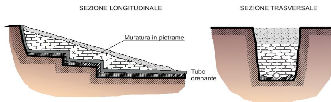
Fig. 43 – Rappresentazione schematica di uno sperone drenante in muratura a secco (da ANPA, 2002).
