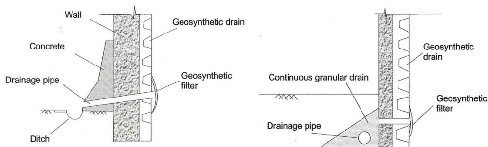
Fig. 48 – Utilizzo dei geosintetici nel drenaggio di strutture di ritenuta, sezioni trasversali (da ORTIGAO & SAYAO, 2004; modificata).
