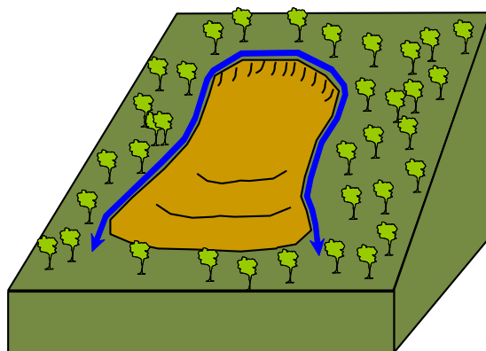
Fig. 37 – Rappresentazione schematica dell'effetto prodotto da un fosso di guardia (porzione sommitale) e di perimetrazione (porzioni laterali) su di un corpo in frana: le acque provenienti dal versante vengono intercettate ed allontanate (in blu) dall'area instabile, evitandone sia gli effetti erosivi associati al ruscellamento superficiale che la potenziale infiltrazione.
