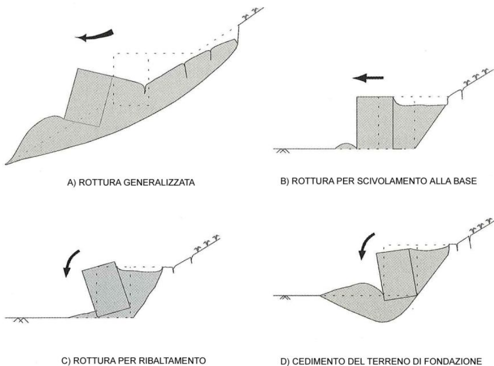
Fig. 51 – Possibili rotture per muri a gravità. Le condizioni prima della rottura per ciascun meccanismo sono riportate in tratteggio (da ORTIGAO & SAYAO, 2004; modificata).
