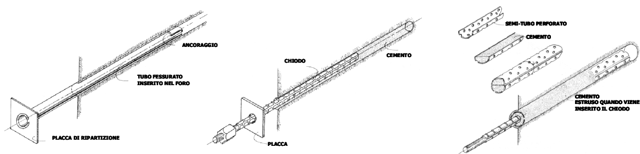
Fig. 85 – Alcune tipologie di chiodi: a sinistra chiodo in acciaio ad ancoraggio puramente attritivo (tubi di ancoraggio); al centro chiodo ad ancoraggio per cementazione; a destra chiodo pefobolt . In quest'ultimo caso l'ancoraggio è ottenuto tramite cemento inserito in tubi forati posizionati entro i fori di chiodatura; l'inserimento della barra provoca l'estrusione del cemento dai fori e l'ancoraggio del chiodo.
