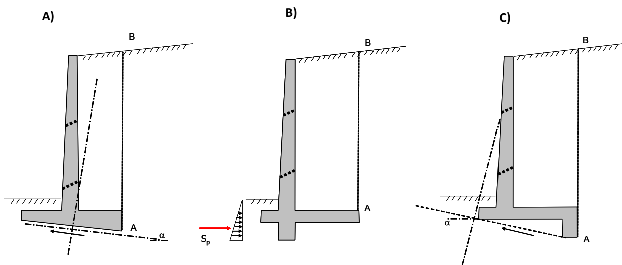
Fig. 68 – Incremento della resistenza allo scivolamento della struttura:
