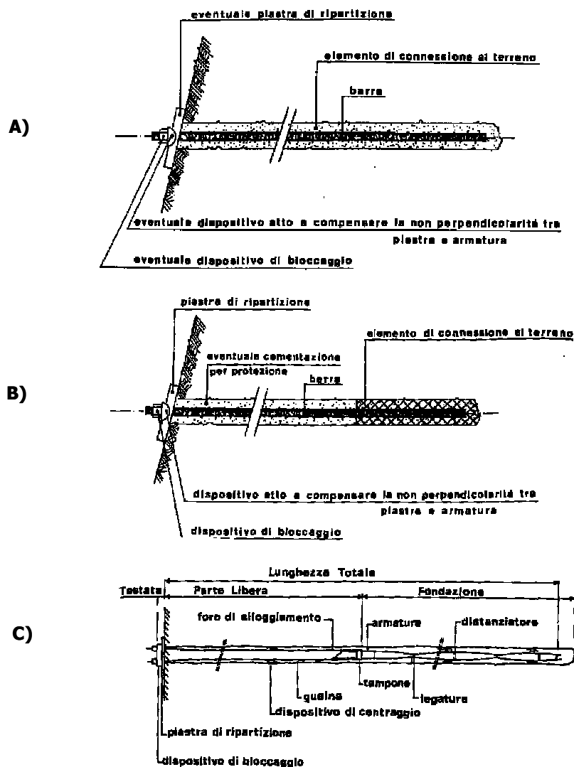
Fig. 84 – Ancoraggi passivi ed attivi. A) chiodo; B) bullone; C) tirante.
