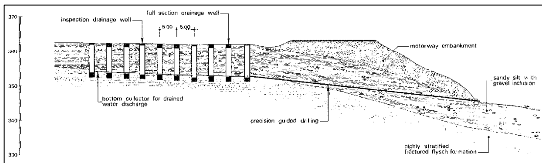
Fig. 51 – Utilizzo di pozzi verticali drenanti lungo il tratto autostradale Firenze – Bologna (da COLLOTTA et al., 1988).
