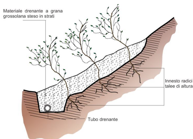
Fig. 40 – Schema di un cuneo drenante. Il materiale drenante è posizionato sulla base del versante dopo averne effettuato una riprofilatura (da ANPA, 2002).
