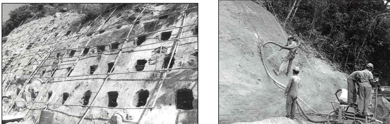
Fig. 91 – Esempi di chiodatura di terreni. A sinistra fase precedente al rivestimento con cemento proiettato; le teste dei chiodi sono alloggiare in nicchie, profonde una ventina di centimetri, scavate nel terreno. A destra fase di rivestimento del versante con cemento proiettato fibrorinforzato SFRS (le immagini sono riprese da ORTIGAO & SAYAO, 2004).
