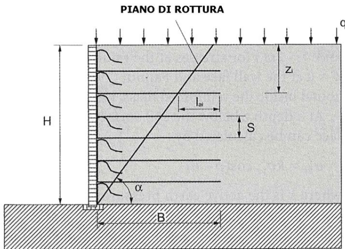
Fig. 100 – Parametri utilizzati per l’analisi della stabilità interna delle terre rinforzate (da ORTIGAO & SAYAO, 2004; modificata).
