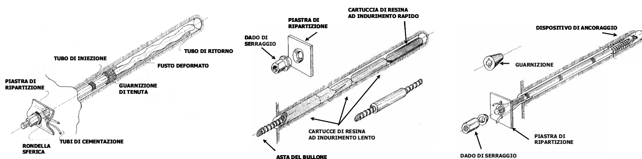
Fig. 86 – Differenti tipologie di bulloni: a sinistra, bulloni ad ancoraggio per cementazione (la porzione terminale del bullone che costituisce l'ancoraggio viene deformata per consentirne il fissaggio fino all'avvenuta presa della malta); al centro, bulloni ad ancoraggio chimico (per evitare problemi di presa anticipata delle resine è necessario che i chiodi non siano eccessivamente lunghi); a destra, bullone ad ancoraggio meccanico.
