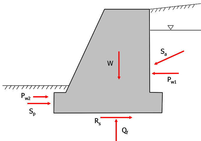
Fig. 50 – Rappresentazione schematica delle forze agenti su di una struttura a gravità.
