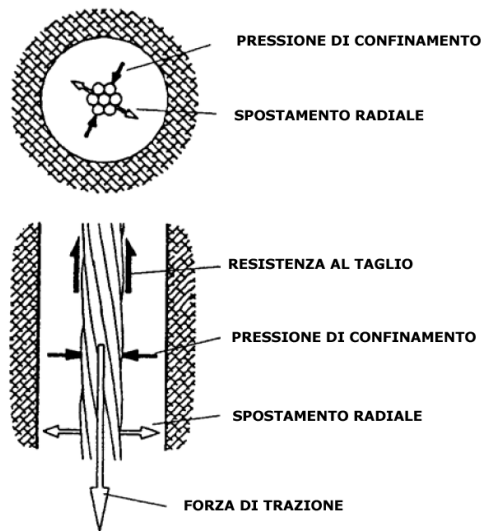
Fig. 87 – A sinistra forze e spostamenti associati con un cavo cementato in foro (da HOEK, 2000; modificato). A destra fase di tesatura di tiranti collocati lungo il cordolo di testa di una paratia di pali di grande diametro.
