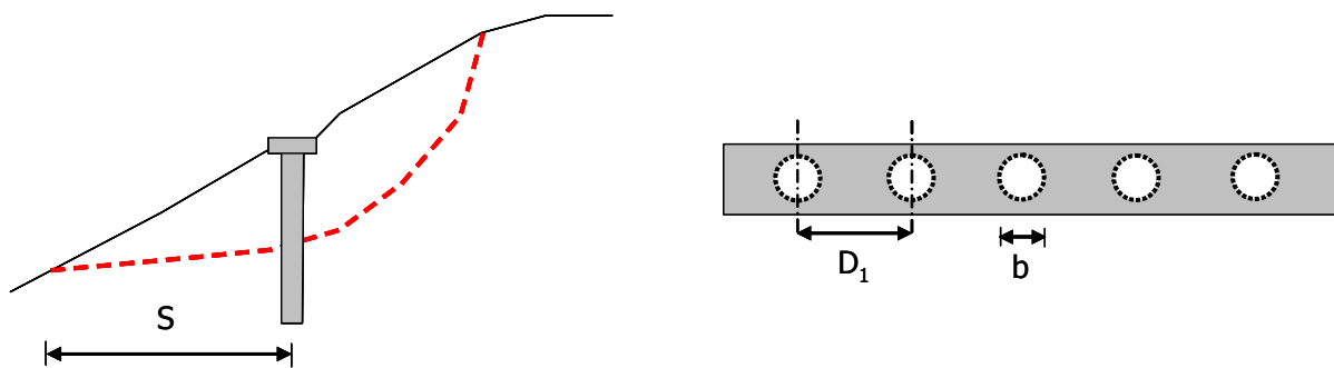
Fig. 80 – Parametri geometrici di una palificata: a sinistra vista in sezione a destra vista in pianta. S = distanza dal piede della frana; D_1 interdistanza tra i pali; b diametro dei pali.
