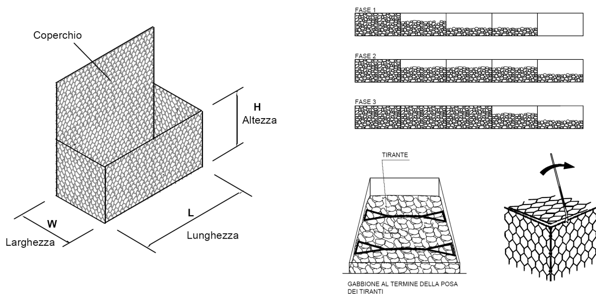
Fig. 60 – A sinistra particolare di un gabbione prima del riempimento; a destra: in alto successive fasi di riempimento della gabbionata, in basso realizzazione dei tiranti sopra ogni strato di pietrame e chiusura del gabbione (schemi ripresi dal catalogo OFFICINE MACCAFERRI S.p.A.).
