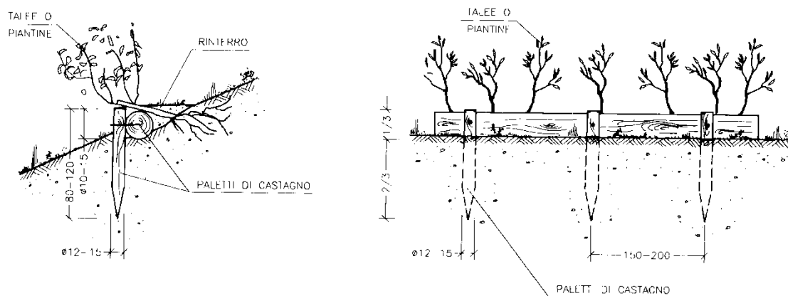
Fig. 27 – Vista in sezione (a sinistra) e frontale (a destra) di una palizzata con un solo ordine di pali trasversali (da REGIONE LIGURIA, 1997).
