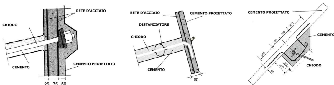
Fig. 92 – Vari sistemi di fissaggio dei chiodi al rivestimento: a sinistra serraggio tramite bulloni; al centro piegatura della testa del chiodo; a destra cementazione della testa del chiodo entro nicchie realizzate nel pendio (da ORTIGAO & SAYAO, 2004; modificato).
