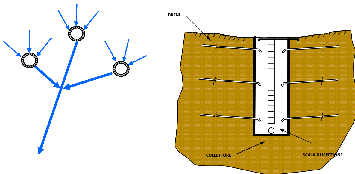
Fig. 49 – Rappresentazione schematica di un sistema di drenaggio profondo attraverso pozzi drenanti e dreni sub-orizzontali. A sinistra vista dall'alto del sistema di drenaggio: le frecce sottili in blu schematizzano dei dreni sub-orizzontali che si dipartono a raggiera dai pozzi; le frecce marcate (sempre in blu) i collettori di fondo per lo scarico delle acque raccolte dai vari pozzi.
