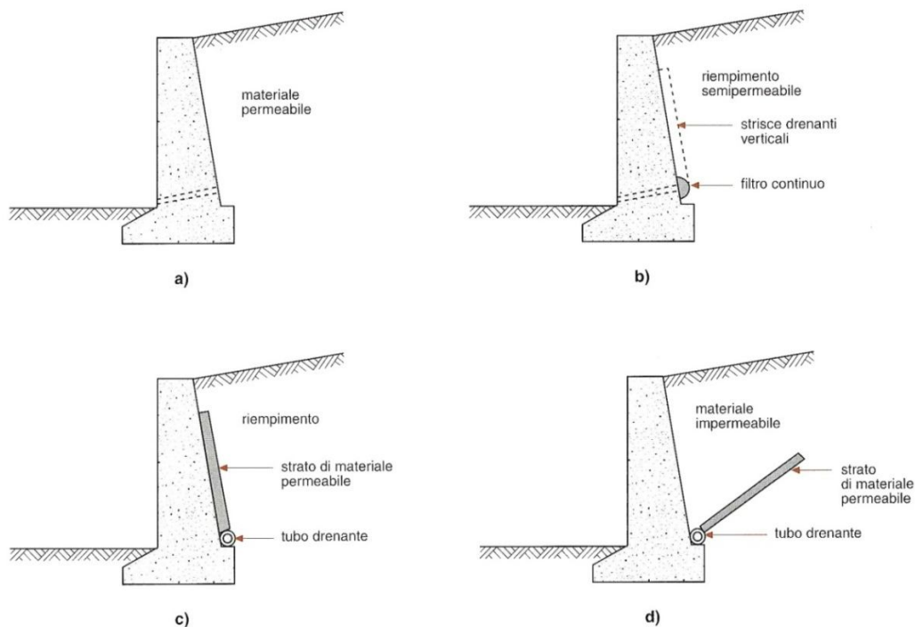
Fig. 59 – Alcuni esempi di sistemi di drenaggio che possono essere utilizzati per lo smaltimento delle acque alle spalle di una struttura di sostegno: a) utilizzo di materiale drenante come riempimento alle spalle del muro; b) sistema di drenaggio utilizzabile nel caso di materiale di riempimento semipermeabile; c) e d) sistema di drenaggio utilizzabile nel caso di riempimento in materiale impermeabile (da COLOMBO et al., 1996).
