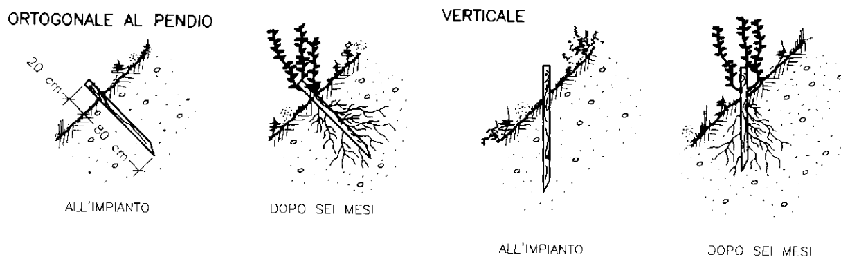
Fig. 18 – Vista in sezione di talee messe a dimora lungo una scarpata (da REGIONE LIGURIA, 1997).
