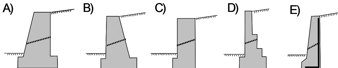
Fig. 58 – Alcune tipologie di muri a gravità: A) muro a gravità con paramento frontale inclinato; B) muro a gravità con paramento posteriore inclinato; C) muro a gravità di forma semplice; D) muro a gravità con paramento posteriore a gradini: in questo caso la stabilità è assicurata, oltre che dal peso della struttura, dal terreno che grava sul tetto dei vari gradini; E) muro a semigravità con rinforzi in acciaio (ad L) nella parte posteriore.
