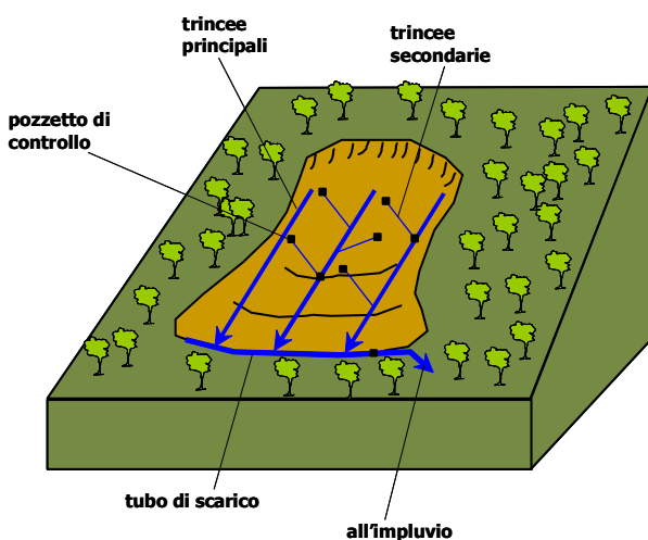
Fig. 41 – Rappresentazione schematica di un intervento di stabilizzazione di un corpo di frana tramite un sistema di trincee drenanti.
