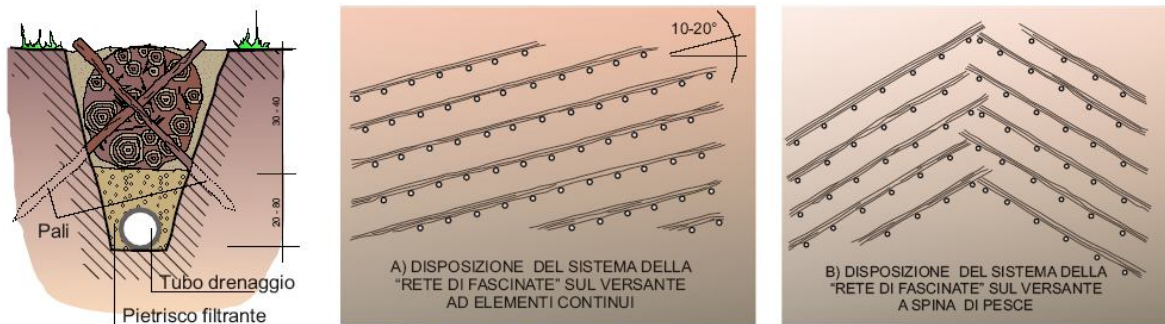
Fig. 24 – Utilizzo delle fascinate come sistemi di drenaggio superficiale. A sinistra sezione tipo di un sistema di drenaggio realizzato con fascine; al centro vista planimetrica di un sistema di fascinate disposte obliquamente rispetto alle curve di livello per evitare ristagni d'acqua; a destra vista planimetrica di un sistema di fascinate disposto a spina di pesce (da ANPA, 2002).
