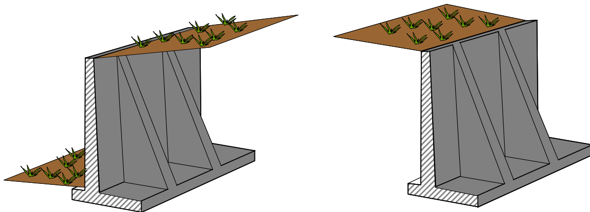
Fig. 70 – Muri a mensola con contrafforte: a sinistra contrafforti posizionati nella porzione interna del muro; a destra contrafforti posizionati nella faccia a vista del muro.
