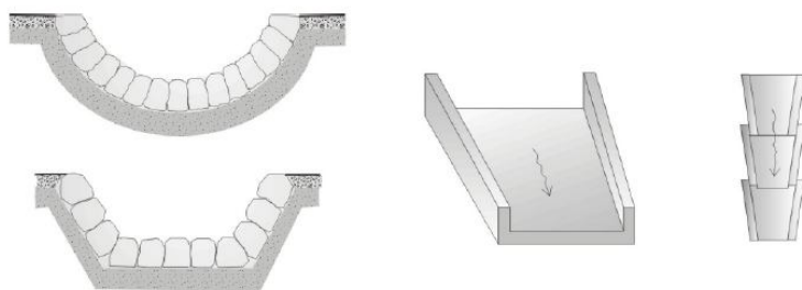
Fig. 35 - Canalette superficiali in pietrame sbozzato, a sinistra, e ad elementi prefabbricati in calcestruzzo a destra (da ANPA, 2002).
