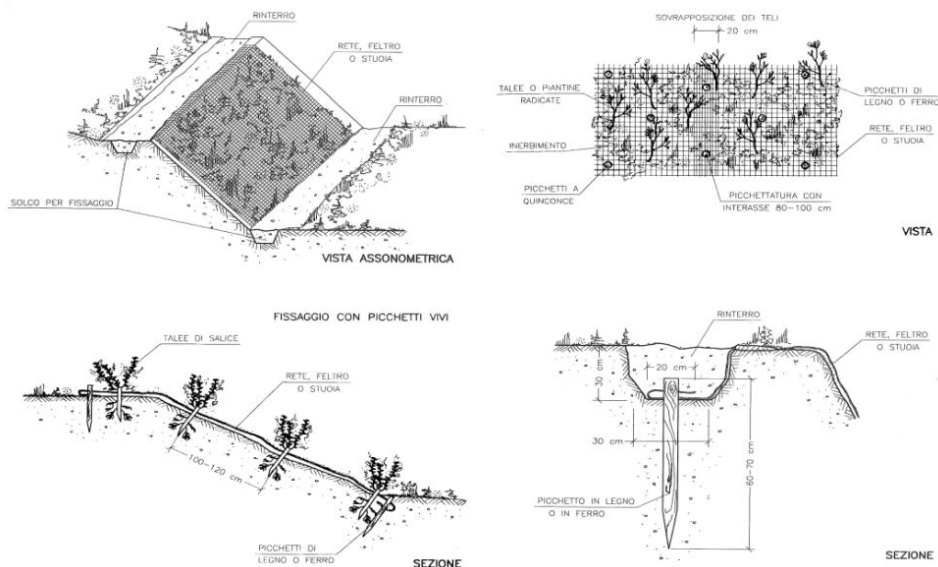
Fig. 13 – Viste esemplificative di un intervento di rivestimento; in basso a destra particolare del picchettamento di monte del rivestimento (da REGIONE LIGURIA, 1997).
