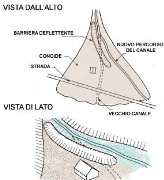
Fig. 112 – Rappresentazione schematica di una barriera deflettente.
