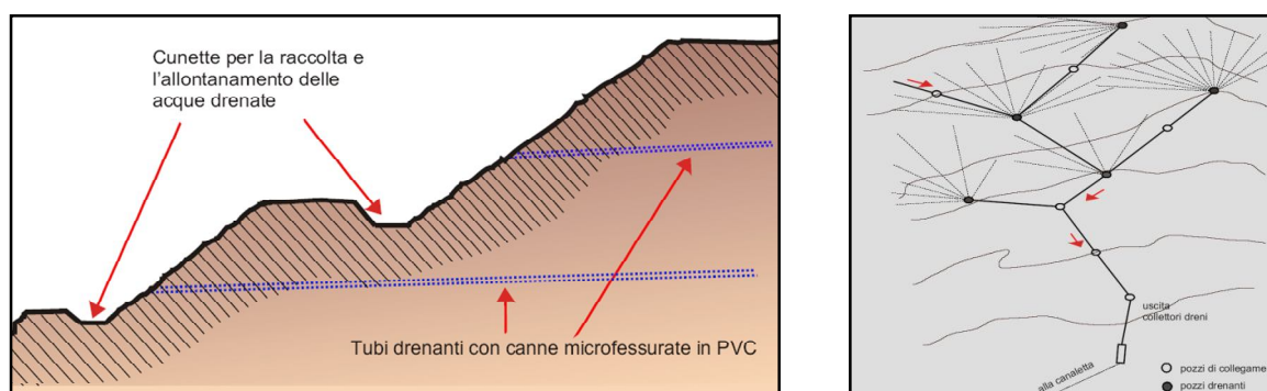
Fig. 46 – Esempi di applicazione di dreni sub-orizzontali: a sinistra reti di dreni sub-orizzontali con scarico delle acque drenate in canalette; a destra sistema di dreni orizzontali distribuiti a raggiera che fanno confluire le acque drenate in pozzetti verticali di grande diametro (da ANPA, 2002; modificato).
