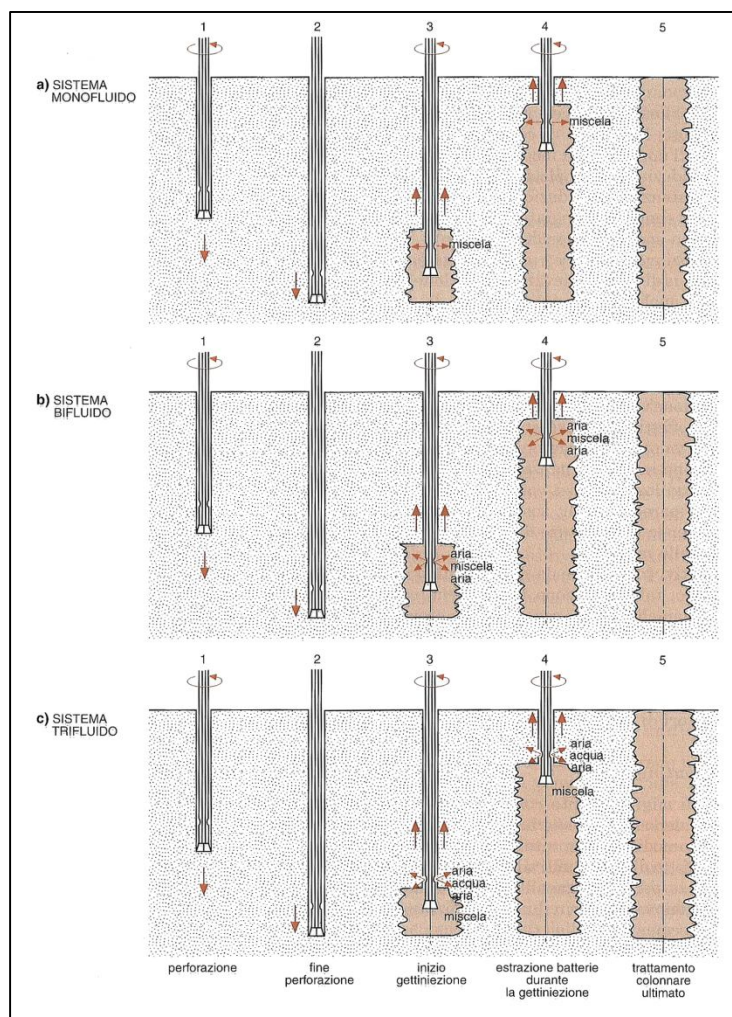
Fig. 103 – Sequenze operative corrispondenti ai differenti sistemi di gettiniezione: a) iniezione della sola miscela cementizia; b) iniezione della miscela cementizia assieme ad aria compressa per aumentare il raggio di azione del trattamento; c) l'azione disagregante è ottenuta grazie a getti coassiali ad alta pressione di acqua ed aria, contemporanei all'iniezione della miscela cementizia (da COLOMBO et al. , 1996).
