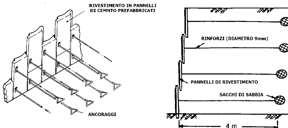
Fig. 99 – Rappresentazioni schematiche di terre ancorate. A sinistra, elementi di ancoraggio ottenuti piegando l'estremità inferiore delle barre a triangolo (da MURRAY & IRWIN, 1981; modificato). A destra, ancoraggi realizzati tramite sacchi di sabbia connessi con gli elementi di rinforzo; le barre e gli ancoraggi sono posizionati nel rilevato durante la costruzione (da FUKUOKA, 1986; modificato).
