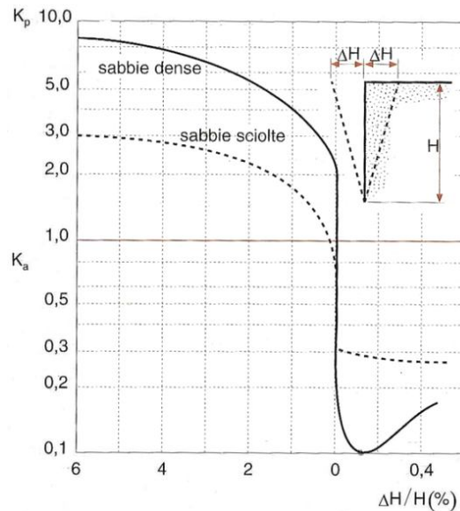
Fig. 54 a – Effetti del movimento di un muro (rotazione del muro \Delta H/H ) sulla spinta del terreno. Il diagramma ripreso da COLOMBO (1996) evidenzia i valori di rotazione del muro necessari per portare a rottura un terreno non coesivo (sia per spinta passiva che attiva). Nel caso di terreni coesivi la differenza tra i valori di rotazione necessari per mobilitare la resistenza passiva e attiva è minore; NAVFAC (1986) riporta per la rottura attiva valori di rotazione compresi tra 1 e 2%, mentre per rottura passiva valori di rotazione compresi tra 2 e 4% -
