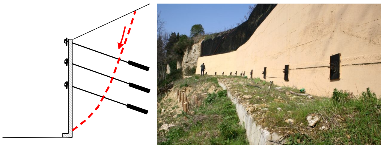
Fig. 81 –A sinistra sezione schematica di un muro tirantato; la linea rossa tratteggiata rappresenta la superficie di scivolamento. A destra muro di sostegno tirantato, realizzato per la stabilizzazione di un versante.
