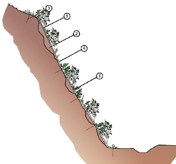
Fig. 33 – Intervento di rivestimento a tasche. 1- rete metallica; 2- terreno di riempimento; 3- chiodatura; 4- stuoia; 5- talea di salice (da ANPA, 2002).
