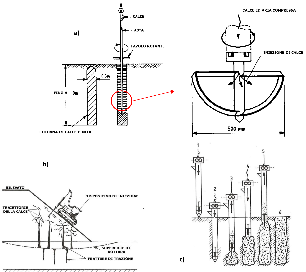
Fig. 104 – Trattamenti chimici del terreno: a) realizzazione di colonne di calce in situ tramite un'apposita attrezzatura in grado di perforare e mescolare il terreno con la soluzione di calce; b) impregnazione delle fratture; c) realizzazione di pali di calce nel terreno (da ROGERS & BRUCE, 1991; modificato).
