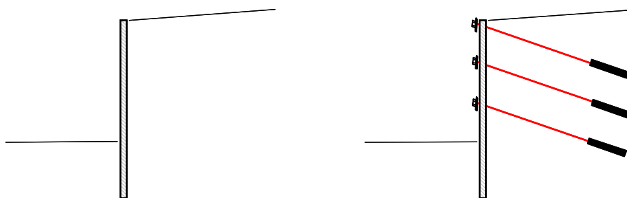
Fig. 71 – Sezione schematica di una paratia: a sinistra senza tiranti, a destra tirantata.
