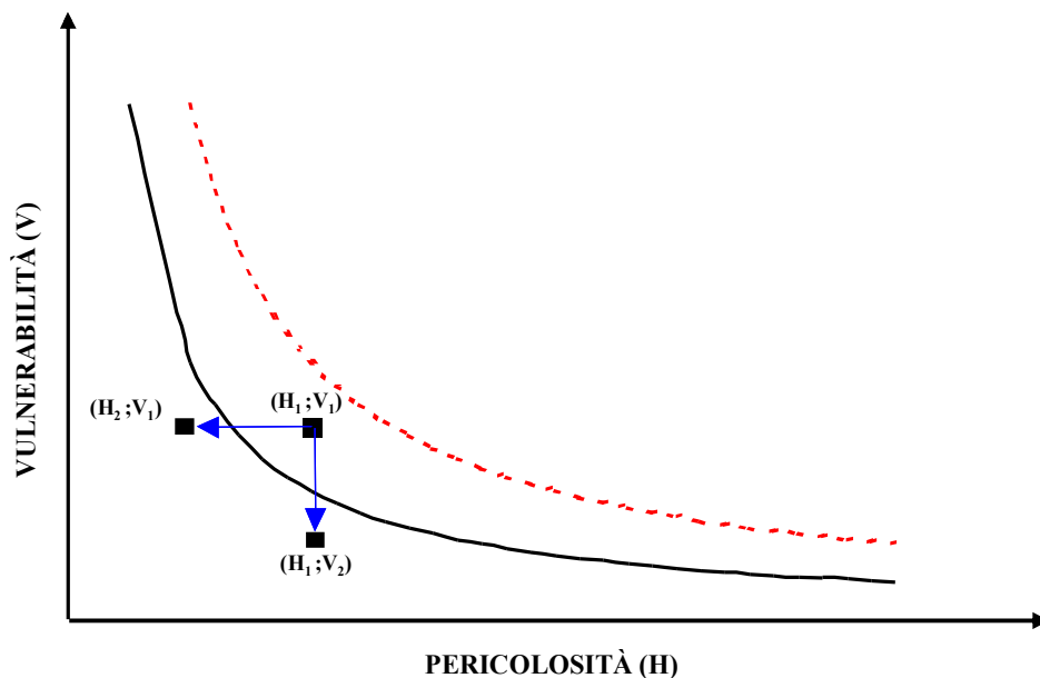
Fig. 1 – Rappresentazione schematica dell'effetto delle differenti strategie di mitigazione del rischio: le curve in nero (continua) ed in rosso (tratteggiata) schematizzano la soglia del rischio accettabile per un dato valore degli elementi a rischio, i vettori in blu le strategie di correzione (vettore orizzontale) e di desensibilizzazione degli elementi a rischio (vettore verticale) .
