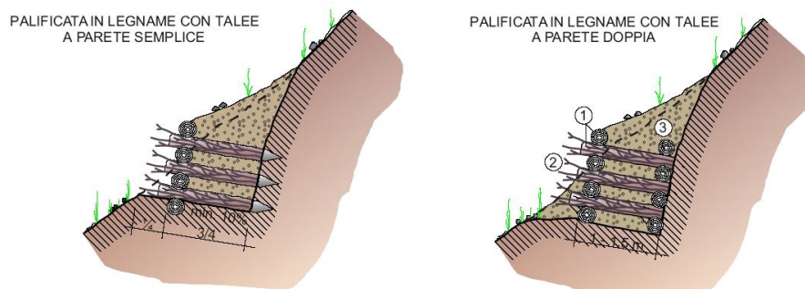
Fig. 30 – Differenti tipologie di palificate. 1- Tondame scortecciato o legname squadrato; 2- ramaglia viva o talee; 3- terreno di riporto (da ANPA, 2002).
