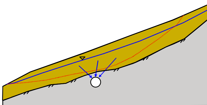
Fig. 53 – Rappresentazione schematica di un sistema di drenaggio profondo attraverso una galleria drenante. La galleria è realizzata parallelamente al versante all'interno del materiale stabile (in grigio); dalla volta si dipartono dreni (in blu) per la dissipazione delle pressioni interstiziali dall'area in frana.
