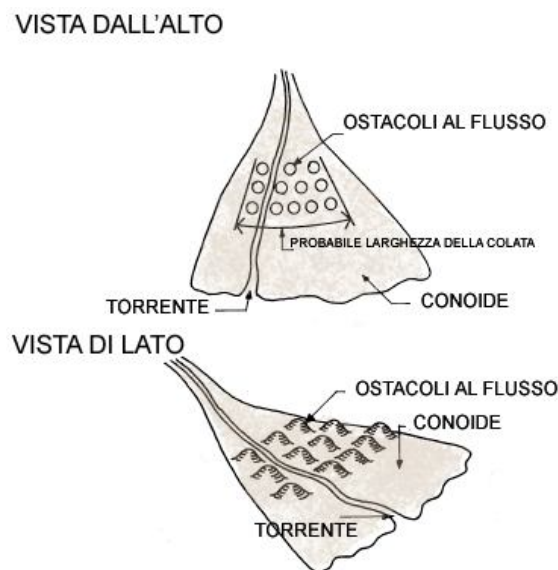
Fig. 108 – Dossi in terra realizzati come ostacolo al flusso entro l'area di deposito.
