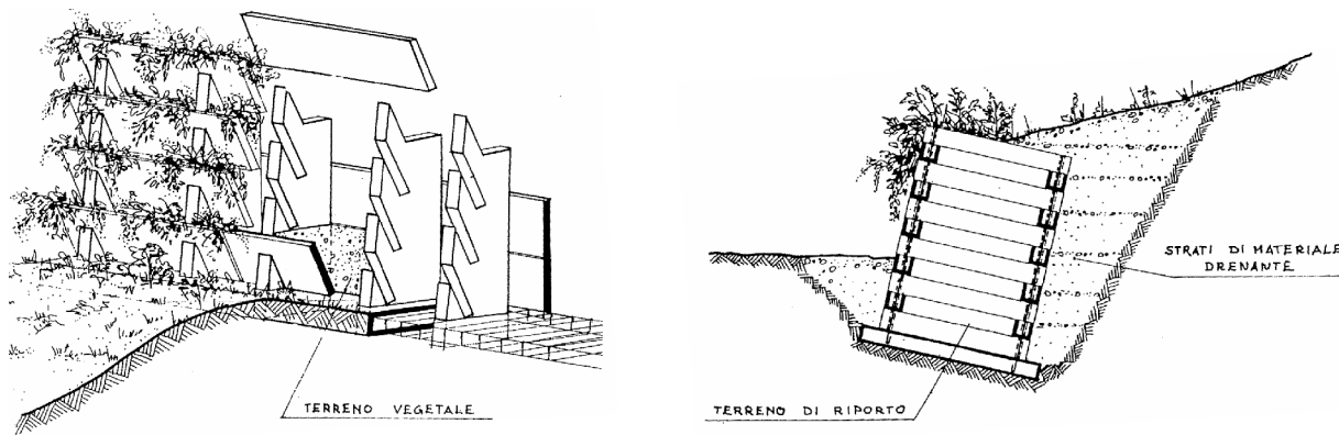
Fig. 65 – Rappresentazioni schematiche di differenti tipologie di muri cellulari: a sinistra muro con elementi planari (pannelli) in calcestruzzo disposti in maniera tale da formare una sorta di scaffalatura riempita con terreno vegetale; a destra sezione tipo di un muro cellulare in travi di calcestruzzo (da REGIONE EMILIA ROMAGNA, 1993).
