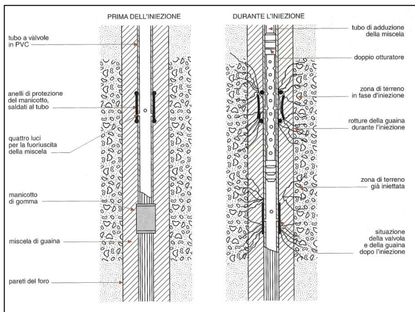
Fig. 102 – Iniezione controllata tramite tubi valvolati (da COLOMBO et al. , 1996).
