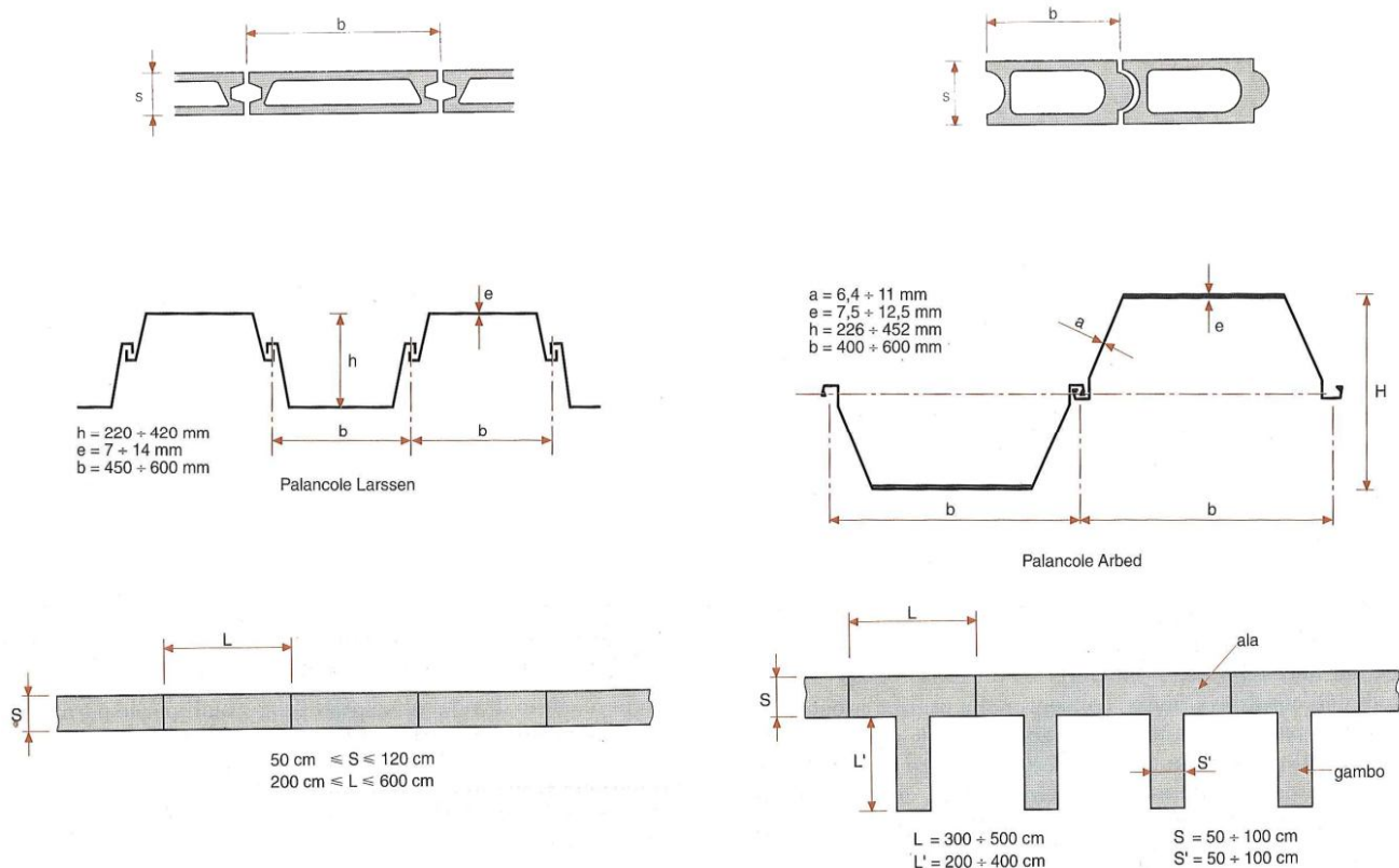
Fig. 72 – Differenti tipologie di paratie utilizzate nel sostegno di scavi. In alto paratie ad elementi prefabbricati in calcestruzzo; dopo la realizzazione di una apposita trincea, si provvede al posizionamento degli elementi ed al successivo scavo del terreno. Al centro paratie metalliche; i vari elementi sono infissi nel terreno prima dello scavo e possono essere lasciati in opera o sfilati, dopo la realizzazione della struttura definitiva di sostegno dello scavo, per poter essere riutilizzati. In basso differenti diaframmi in cemento armato gettati in opera; quest'ultima tipologia di paratia è utilizzata per il sostegno di scavi di maggiori larghezze (da COLOMBO et al., 1996).
