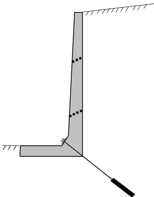
Fig. 69 – Muro in cemento armato (a mensola con sezione ad L) con base tirantata; in tratteggio i dreni del muro; i tiranti sono descritti tra le strutture di rinforzo interno (interventi D1a).
