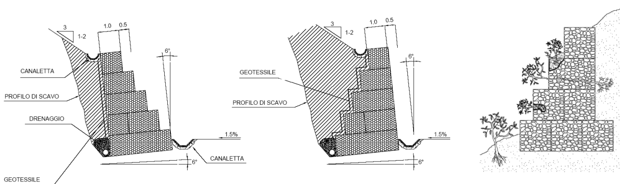
Fig. 61 – Differenti tipologie di gabbionate: a sinistra muro a gradoni esterni, al centro muro a gradoni interni; nei due schemi sono riportati anche i sistemi di allontanamento delle acque dalla struttura. A destra muro a gradoni esterni e scarpa interna accoppiato ad interventi di rinverdimento; le talee possono essere messe in posa nei gabbioni, interrompendo il riempimento in pietrame, oppure tra un gabbione e l'altro (schemi ripresi dal catalogo OFFICINE MACCAFERRI S.p.A.).
