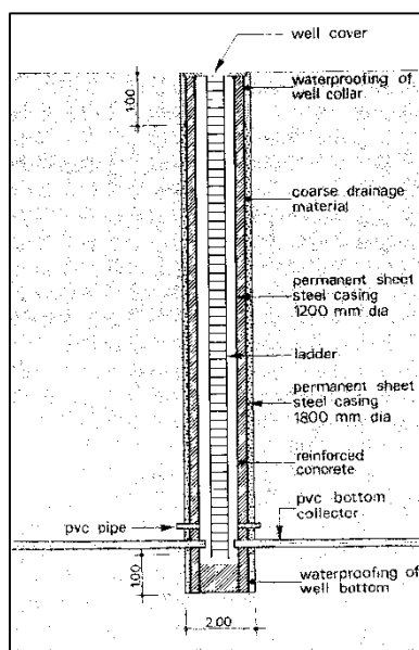
Fig. 52 – Schema di un pozzo drenante di ispezione avente anche una funzione strutturale (da COLLOTTA et al., 1988).
