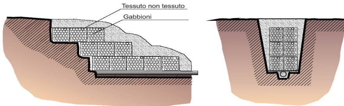
Fig. 44 – Rappresentazione schematica di uno sperone drenante in gabbioni (da ANPA, 2002).
