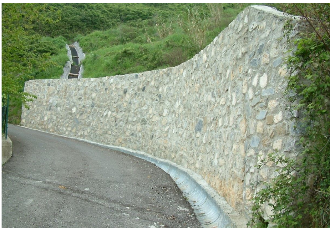
Fig. 57 - Muro di sostegno in calcestruzzo, rivestito con muratura in pietra.
