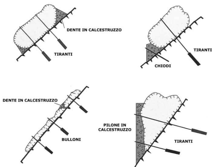
Fig. 90 – Esempi di applicazioni di chiodi, bulloni e tiranti nella stabilizzazione di masse rocciose di varie dimensioni (da ORTIGAO & SAYAO, 2004; modificata).
