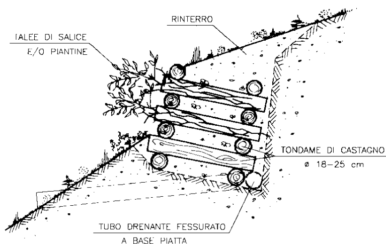
Fig. 31 – Messa in posto di tubi drenanti per l'allontanamento delle acque che si raccolgono alla base delle palificate (da REGIONE LIGURIA, 1997).
