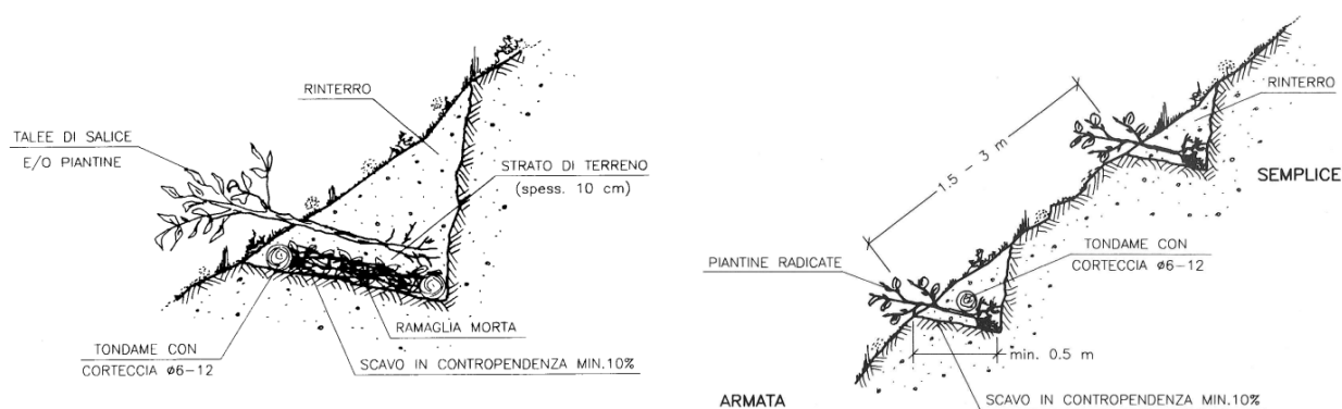
Fig. 21 – Rappresentazione schematica di alcuni tipi di gradonatura. A sinistra vista in sezione di una cordonata; a destra gradonata con piantine, semplice nella parte superiore, armata con tondame nella parte inferiore (da, REGIONE LIGURIA, 1997).
