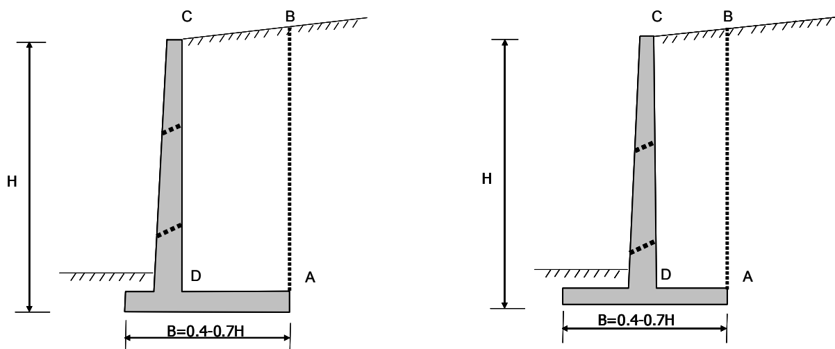
Fig. 67 – Principali tipologie di muri a mensola: a sinistra muro ad L e a destra muro a T rovescia; le linee tratteggiate rappresentano i dreni sulla porzione verticale del muro.
