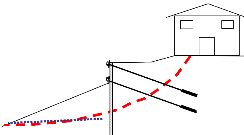
Fig. 74 – Esempio di sistemazione di corpo di frana tramite l'utilizzo di una paratia tirantata. La porzione a valle della paratia è stabilizzata tramite l'uso di dreni suborizzontali (linea tratteggiata in blu).
