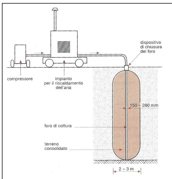
Fig. 105 – Dispositivo per il trattamento termico del terreno a circolazione forzata (da COLOMBO et al. , 1996).
