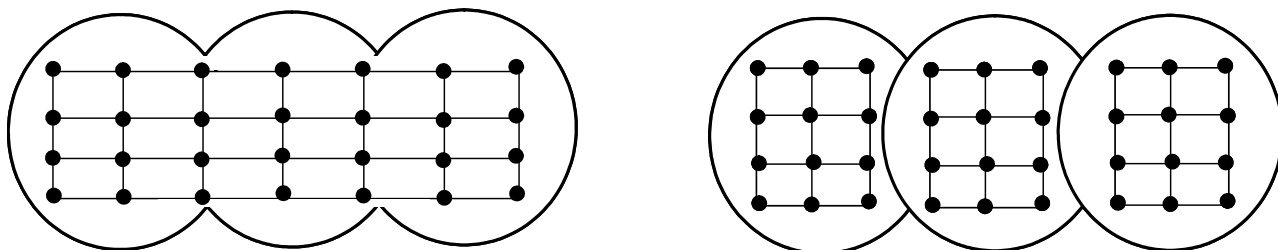
Fig. 79 – Vista in pianta di un diaframma di pali secanti in terreni stabili a sinistra ed in terreni instabili a destra; i reticoli rappresentano l'armatura del diaframma.
