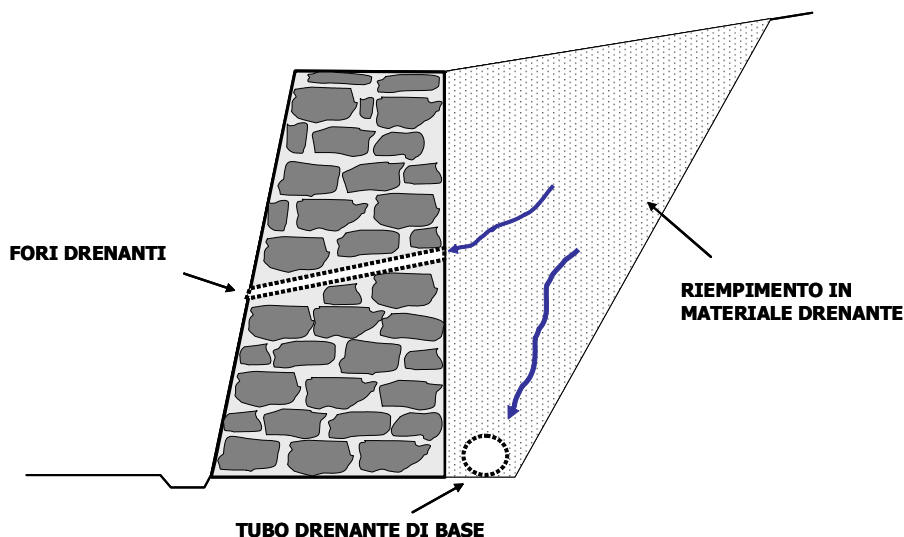
Fig. 55 – Rappresentazione schematica del sistema di drenaggio alle spalle di un muro in muratura. L'acqua alle spalle della struttura percola attraverso il materiale drenante di riempimento e viene allontanata tramite i fori e le feritoie sulla parete del muro e tramite il tubo drenante alla base della struttura.
