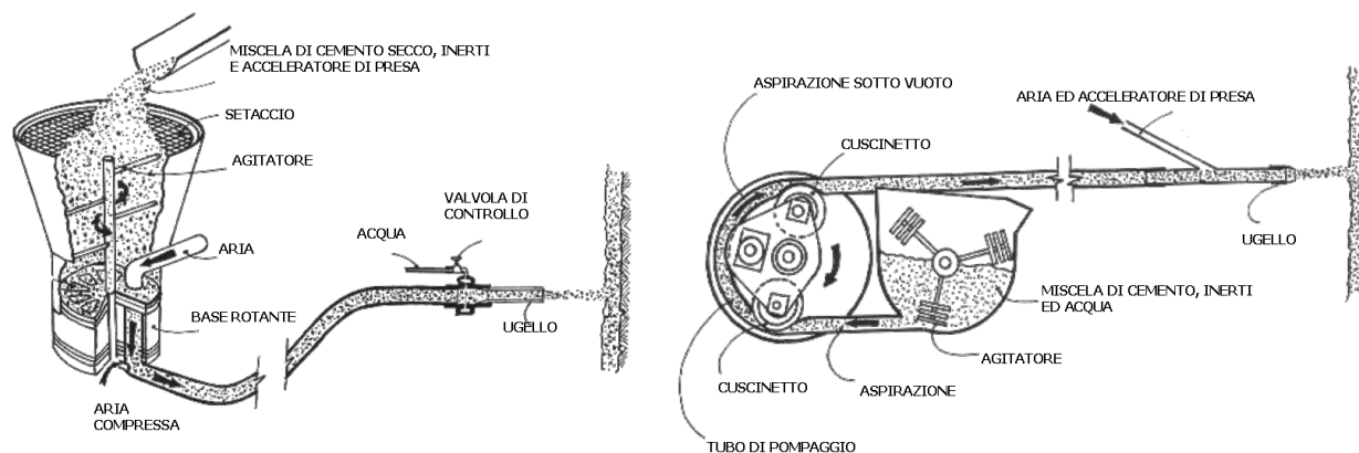
Fig. 96 – Dispositivi utilizzati per l'applicazione del cemento proiettato: miscelazione a secco a sinistra e umida a destra (da HOEK, 2000; modificato).
