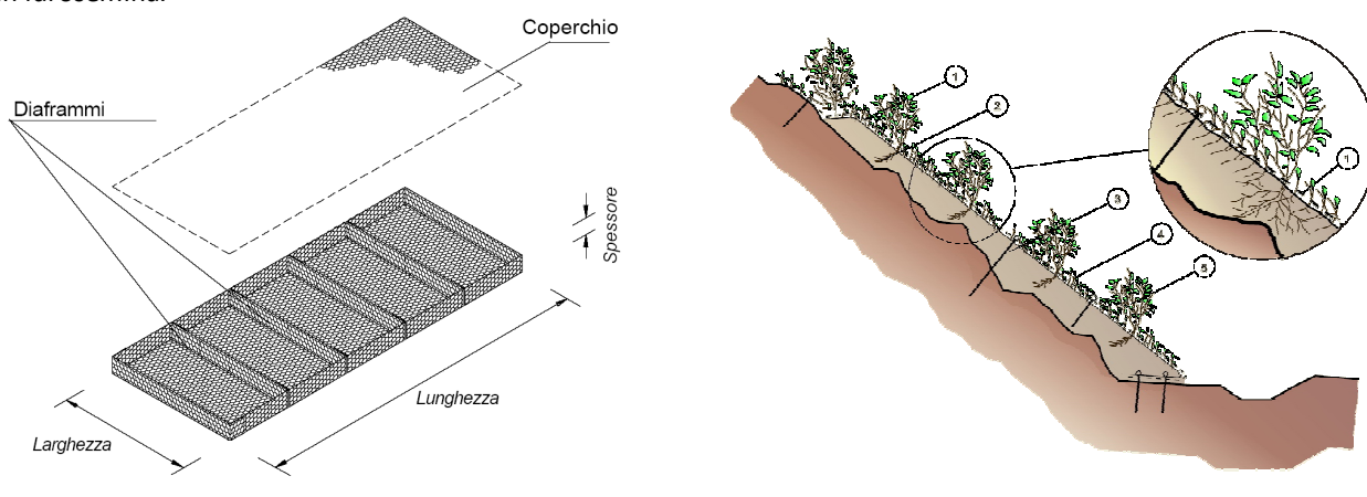
Fig. 34 – Rivestimento tramite materassi prefabbricati. A sinistra un materasso di tipo Reno; a destra un materasso posizionato su di una scarpata: 1- rete metallica; 2- terreno di riempimento; 3- chiodatura; 4- stuoia; 5- talea di salice.
