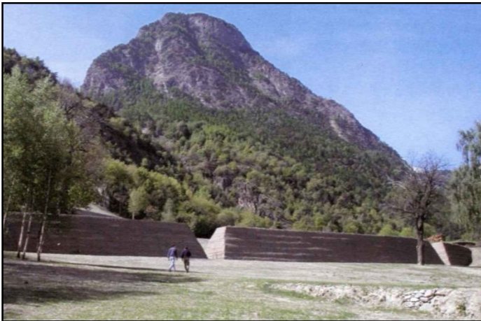
Fig. 116 – Vista da valle di una barriera terminale.
