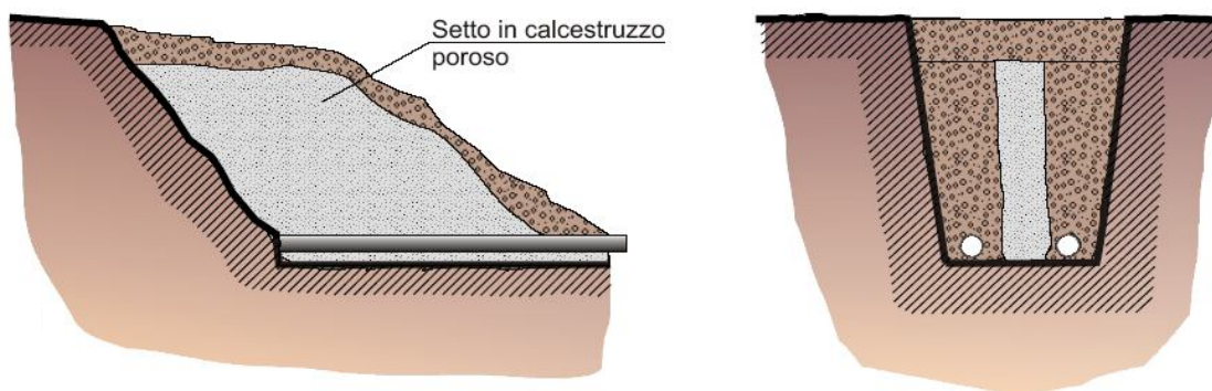
Fig. 45 – Rappresentazione schematica di uno sperone drenante con setto centrale in calcestruzzo poroso (da ANPA, 2002).
