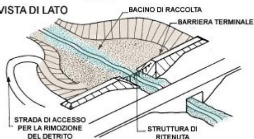
Fig. 119 – Rappresentazione schematica di una diga aperta.
