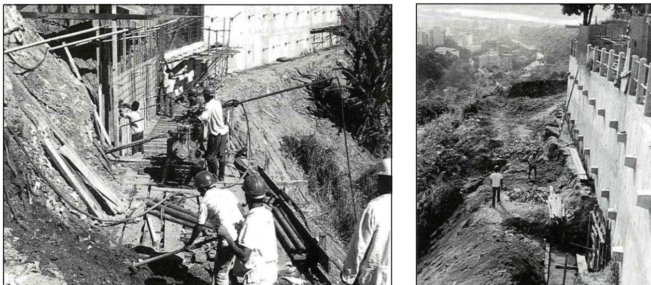
Fig. 82 – Fasi costruttive di muri tirantati. A sinistra muro costruito dal basso verso l'alto: in primo piano fasi di installazione dei tiranti, sullo sfondo posizionamento dell'armatura e muro gettato. A destra muro costruito dall'alto verso il basso: si nota in basso una nicchia scavata e armata; per assicurare la stabilità lo scavo viene effettuato per porzioni limitate, che vengono armate e gettate prima di scavare la porzione limitrofa (da ORTIGAO & SAYAO, 2004).
