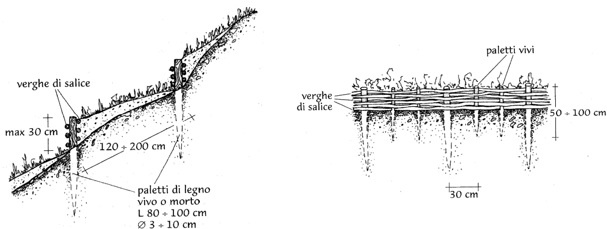
Fig. 25 – Vista in sezione (a sinistra) e frontale (a destra) di una viminata (da PROVINCIA DI TERNI, 2003; modificata).
